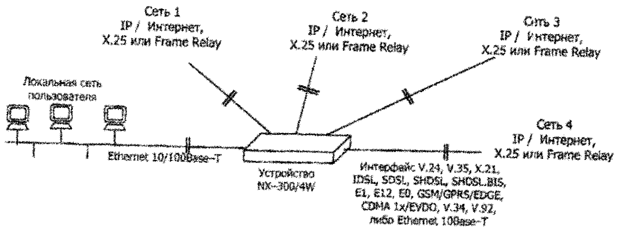
Схема подключения оборудования к сети общего пользования
