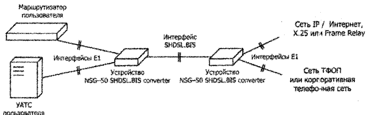
Схема подключения оборудования к сети общего пользования
