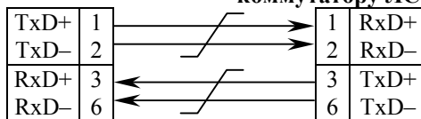
Кабель "Ethernet RJ-45 straight"
