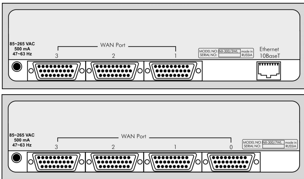
Задняя панель устройств NX-300/3WL (вверху) и NX-300/4W (внизу)
