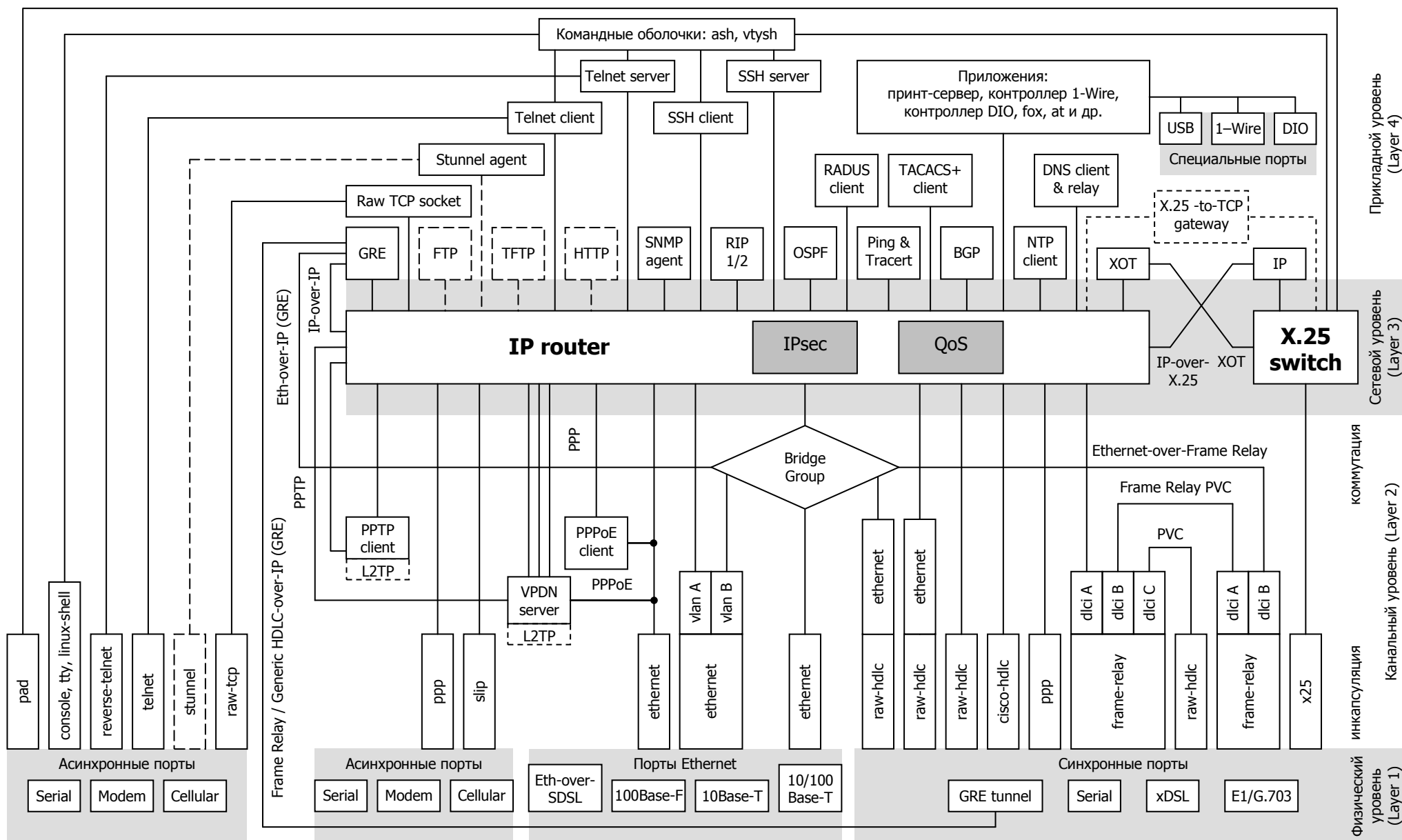
Иерархическая архитектура протоколов передачи данных в NSG Linux
