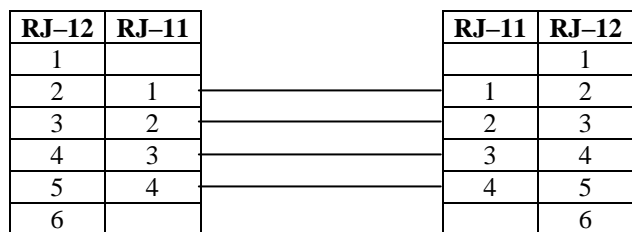
Схема соединительного кабеля
