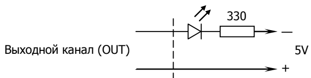
Включение светодиодной индикации
