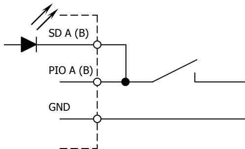
Контроль "сухих контактов" с индикацией
