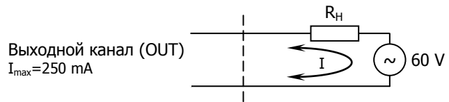
Подключение нагрузки
