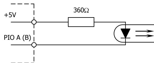
Управление светодиодным индикатором или оптронным ключом
