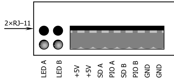
Вид со стороны лицевой панели
