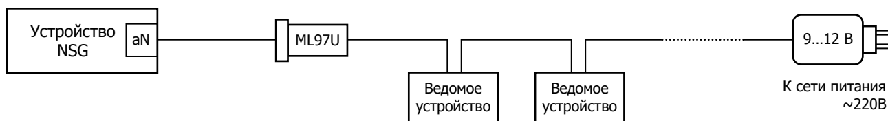
Схема подключения
