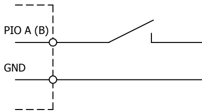
Контроль "сухих контактов" без индикации
