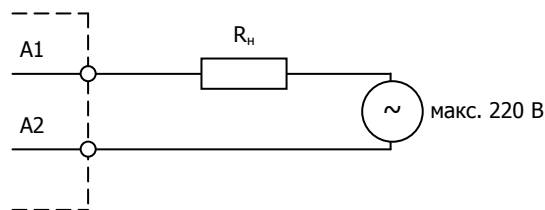
Схемы подключения
