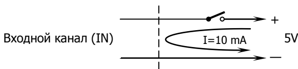
Контроль за "сухими контактами"
