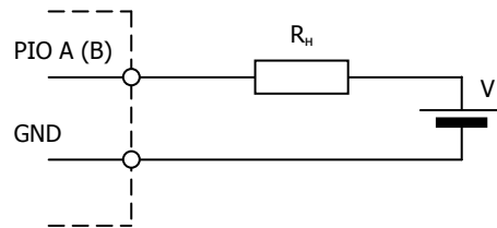
Управление электрической цепью J_{max} = 20 \text{ мА} V_{max} = 28 \text{ В} гальваническая связь
