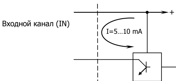
Контроль электрических цепей TTL-уровня
