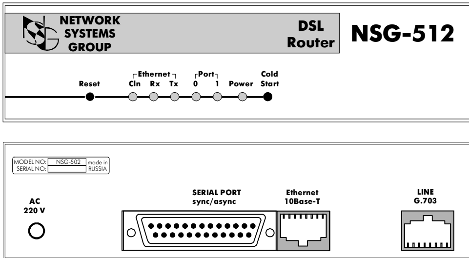
Рис.2 Передняя и задняя панели устройства NSG-512
